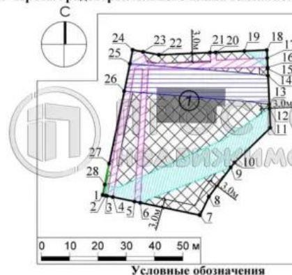
1. Чертеж градостроительного плана земельного участка
